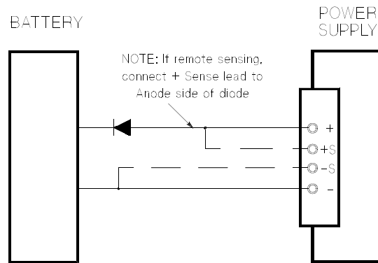
図 3-1. 蓄電池の充電に推奨される保護回路
