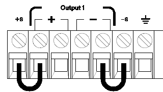
図 2-2. ローカル検出の接続
