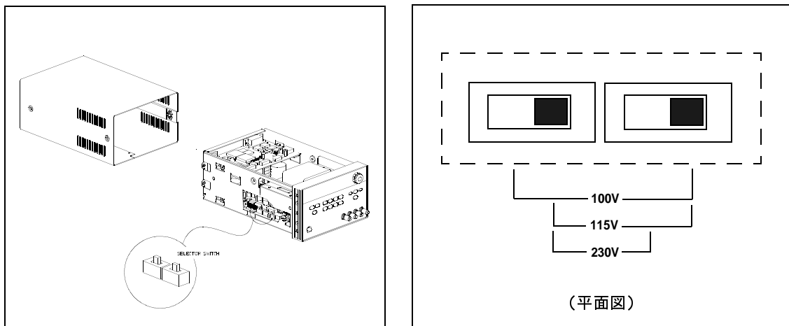
図 1-1. 電源電圧セレクトタ (AC 115V 用)
