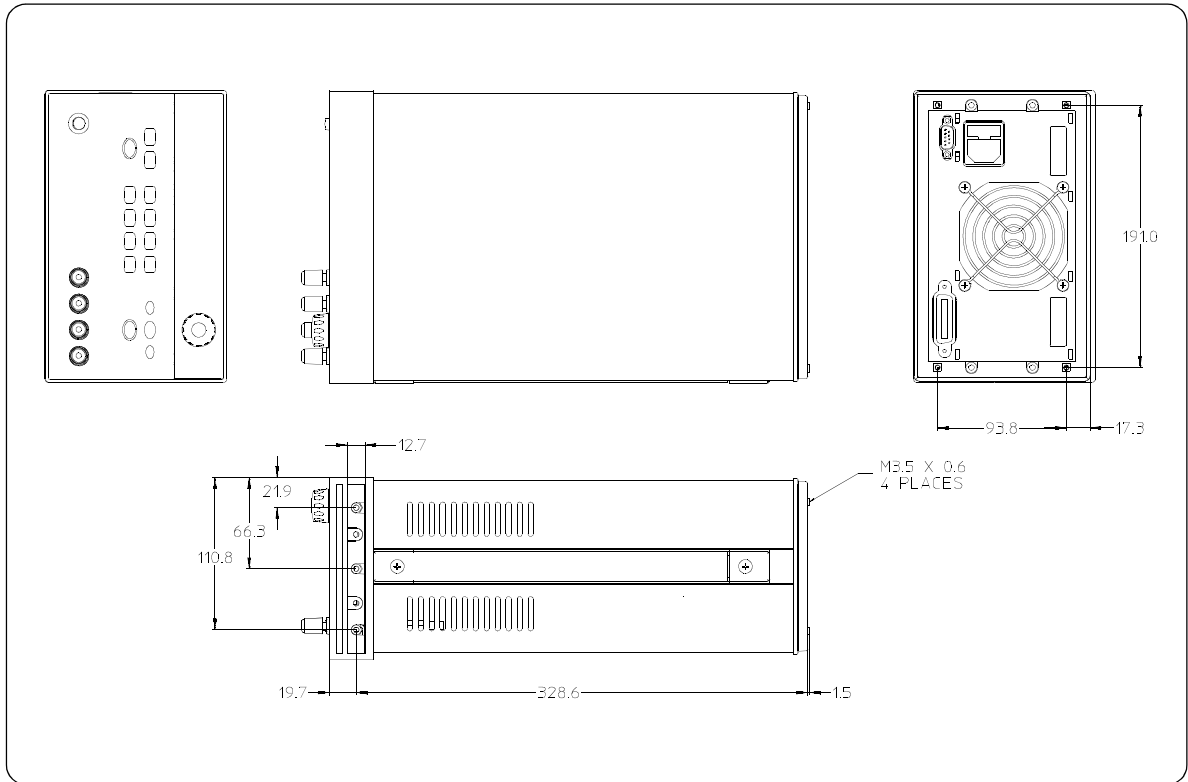
図 8-2. ラック設置寸法
