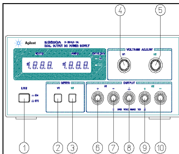
图 2 前面板控制器和指示灯
